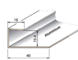
Abschlussprofil Aluminium 8236
